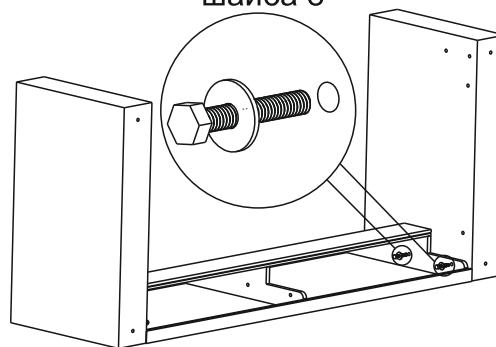
опора шпилька М8х50
